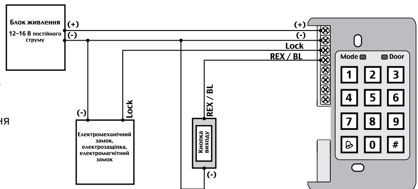
типова схема з'єднання
